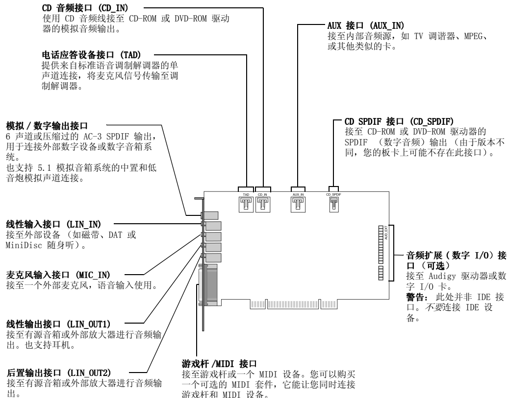
图 1-2: Sound Blaster Audigy (非 SB 1394) 卡上的接口和端口。
