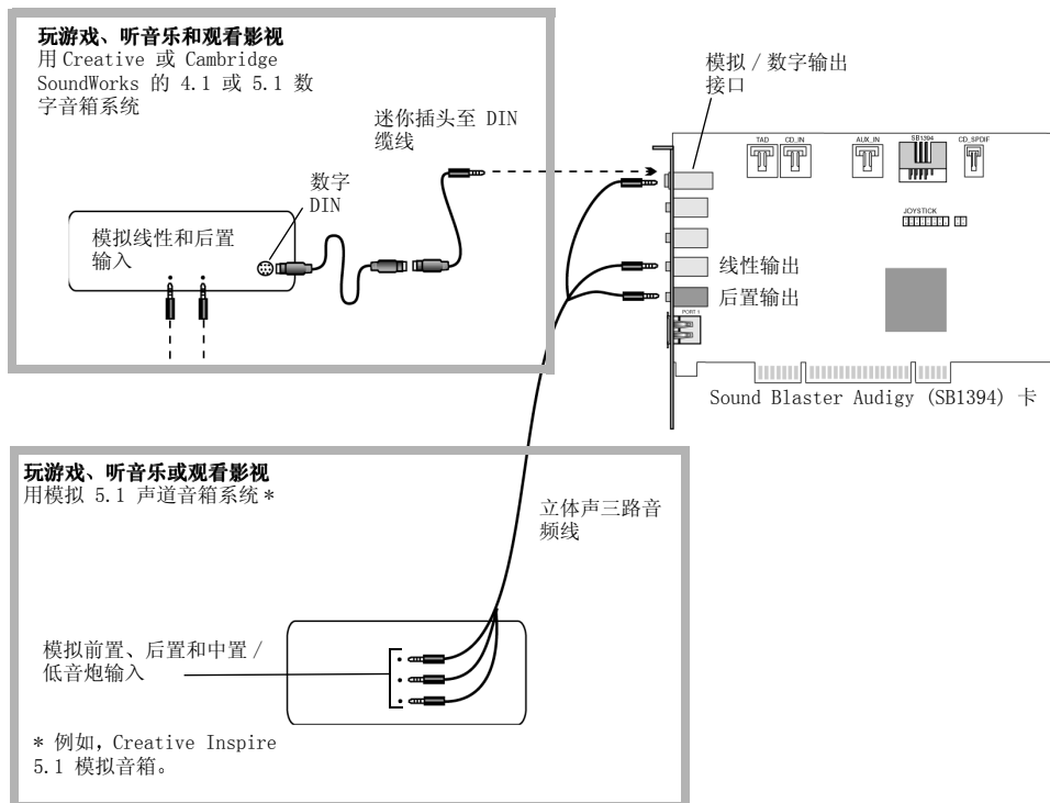
图 1-9: 将 Sound Blaster Audigy (SB1394) 卡接至音箱系统。
