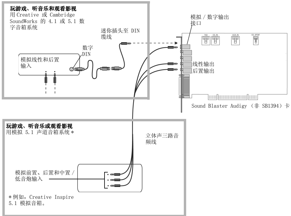
图 1-10: 将 Sound Blaster Audigy (非 SB1394) 卡接至音箱系统。
