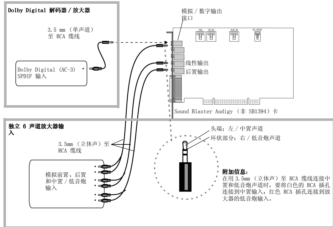
图 1-12: 将外部家用设备接至 Sound Blaster Audigy (非 SB1394) 卡。
