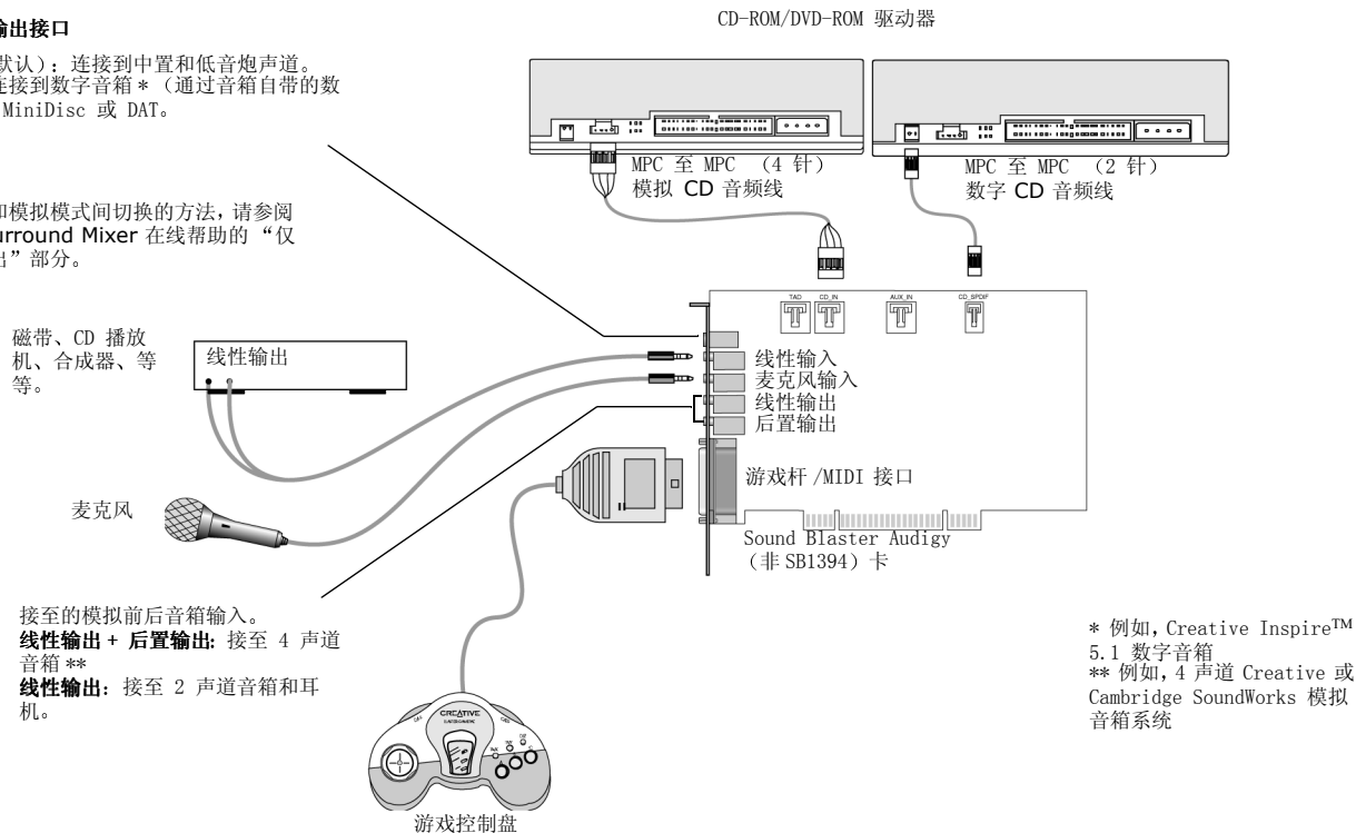
图 1-8: 将其它设备接至 Sound Blaster Audigy (非 SB1394) 卡。
