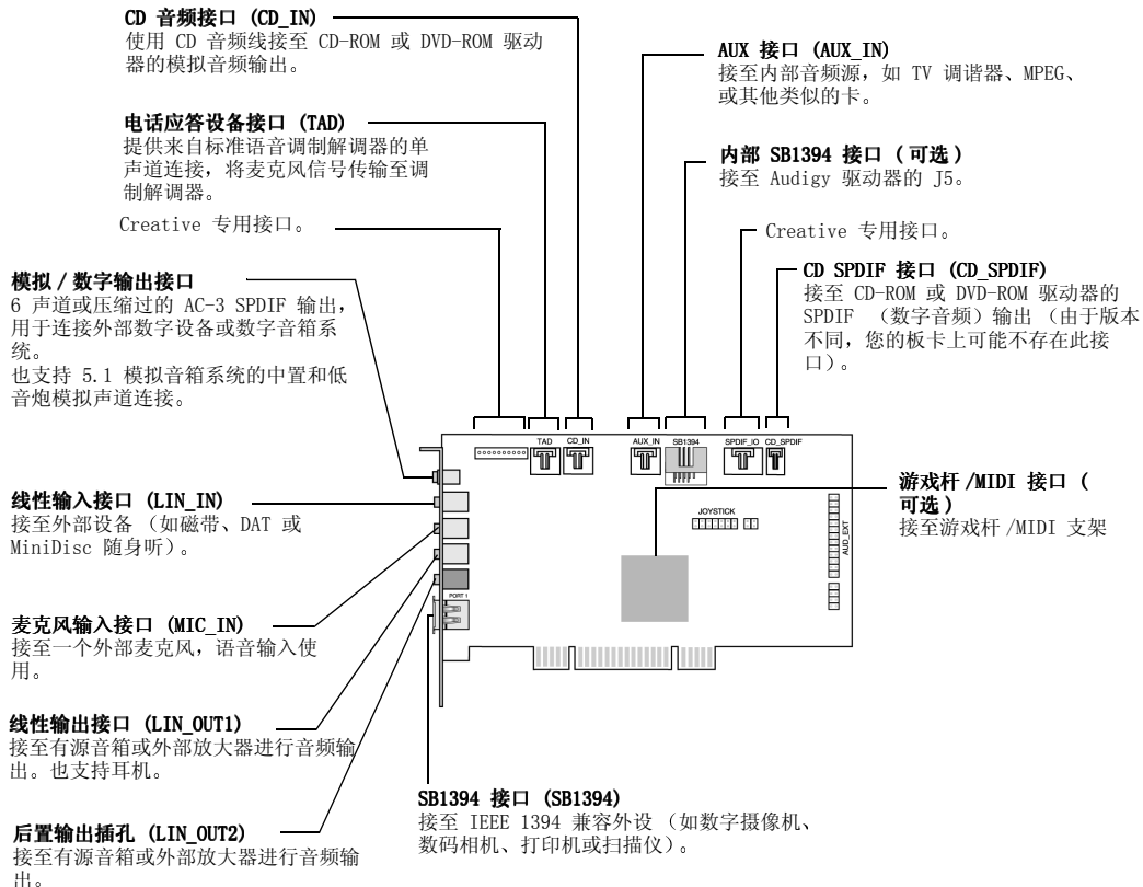
图 1-1: Sound Blaster Audigy (SB1394) 卡上的接口和端口。
