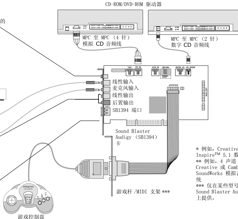
图 1-7: 将其它设备接至 Sound Blaster Audigy (SB1394) 卡。
