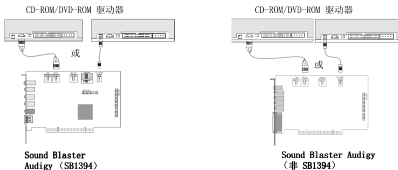
图 1-6: 连接驱动器。
