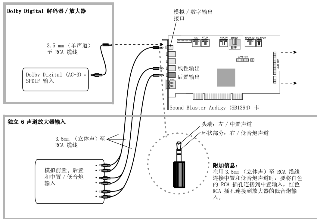
图 1-11: 将外部家用设备接至 Sound Blaster Audigy (SB1394) 卡。
