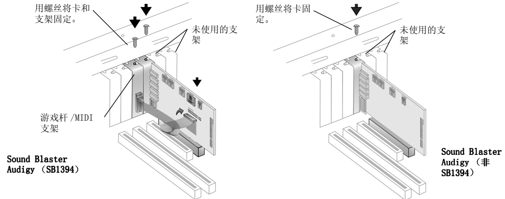
图 1-5: 将声卡固定在扩展槽内。
