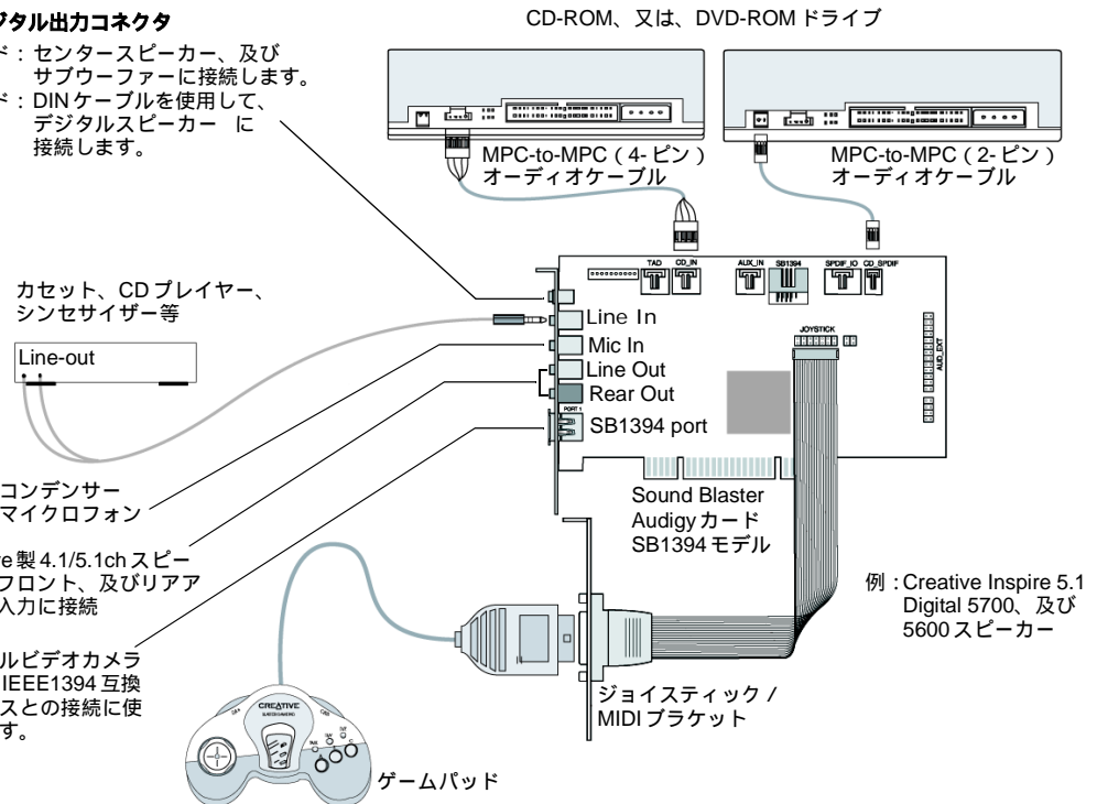
図 1-7 Sound Blaster Audigy カード SB1394 モデルとその他の機器の接続
