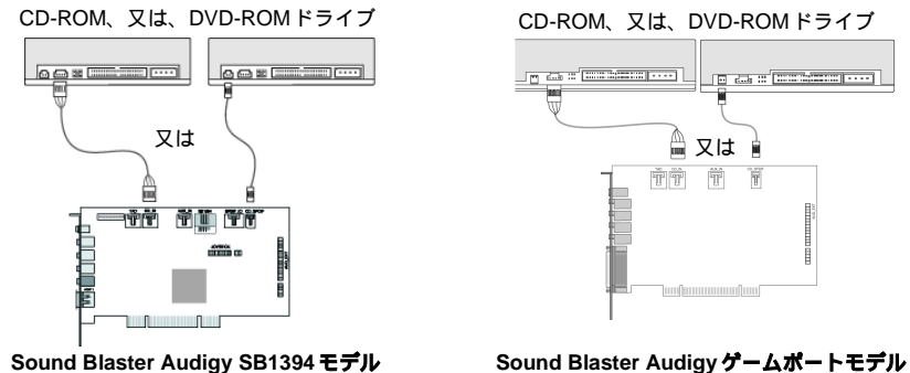
図 1-6 ドライブの接続
