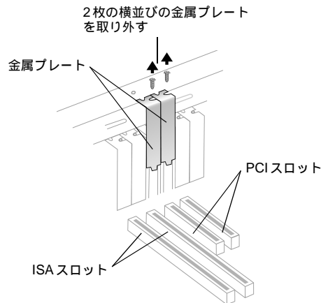
図 1-4 金属プレートの取り外し
