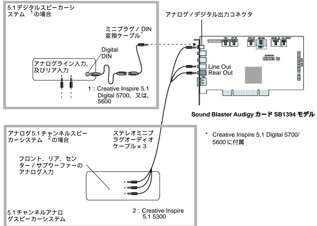
図 1-9 Sound Blaster Audigy カード SB1394 モデルとスピーカーシステムの接続
