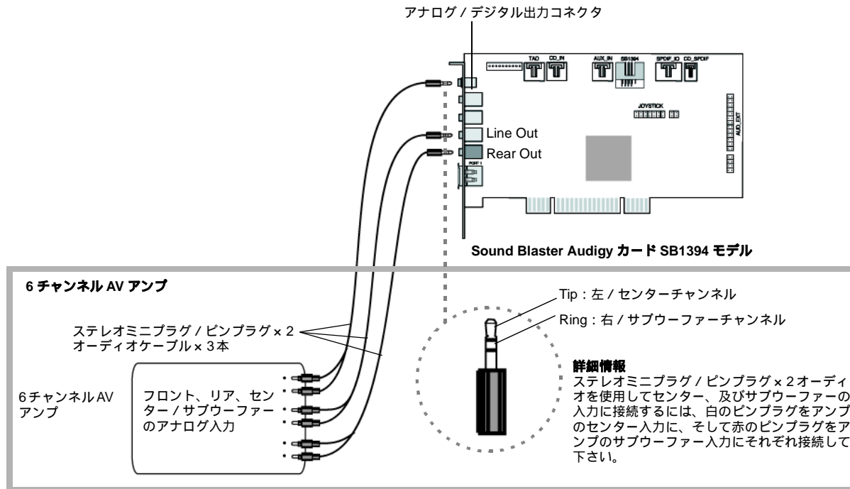
図 1-11 Sound Blaster Audigy カード SB1394 モデルと 6 チャンネル AV アンプとの接続
