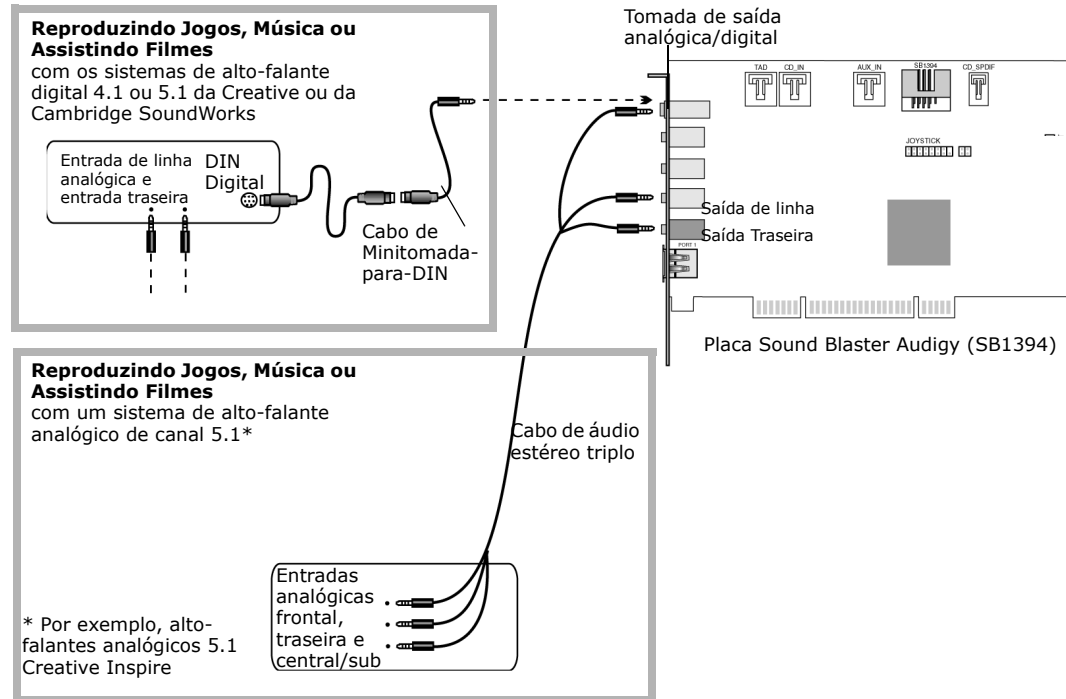
Figura 1-9: Conectando os sistemas de alto-falantes à placa Sound Blaster Audigy (SB1394).
