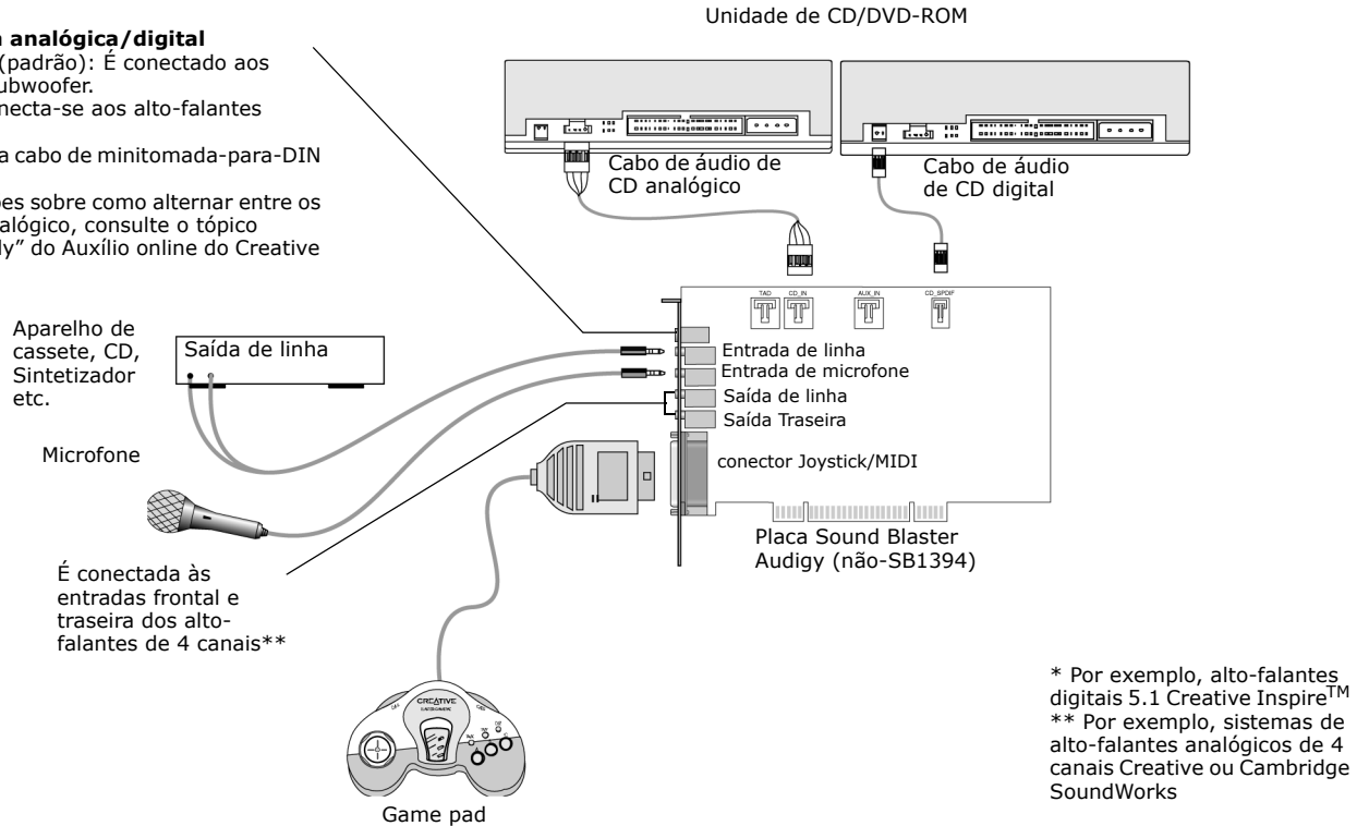
Figura 1-8: Conectando outros dispositivos ao placa Sound Blaster Audigy (não-SB1394).
