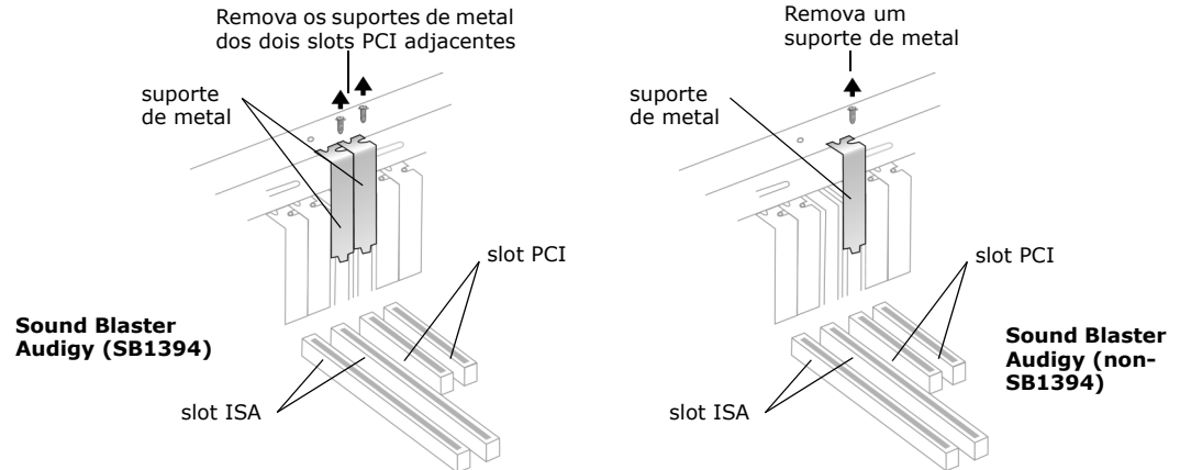
Figura 1-4: Remoção dos suportes de metal.
