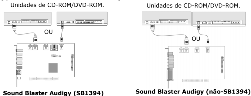
Figura 1-6: Conectando os cabos de áudio analógico/digital às unidades de CD-ROM/DVD-ROM.
