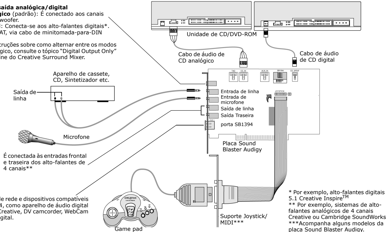
Figura 1-7: Conectando outros dispositivos ao placa Sound Blaster Audigy (SB1394).
