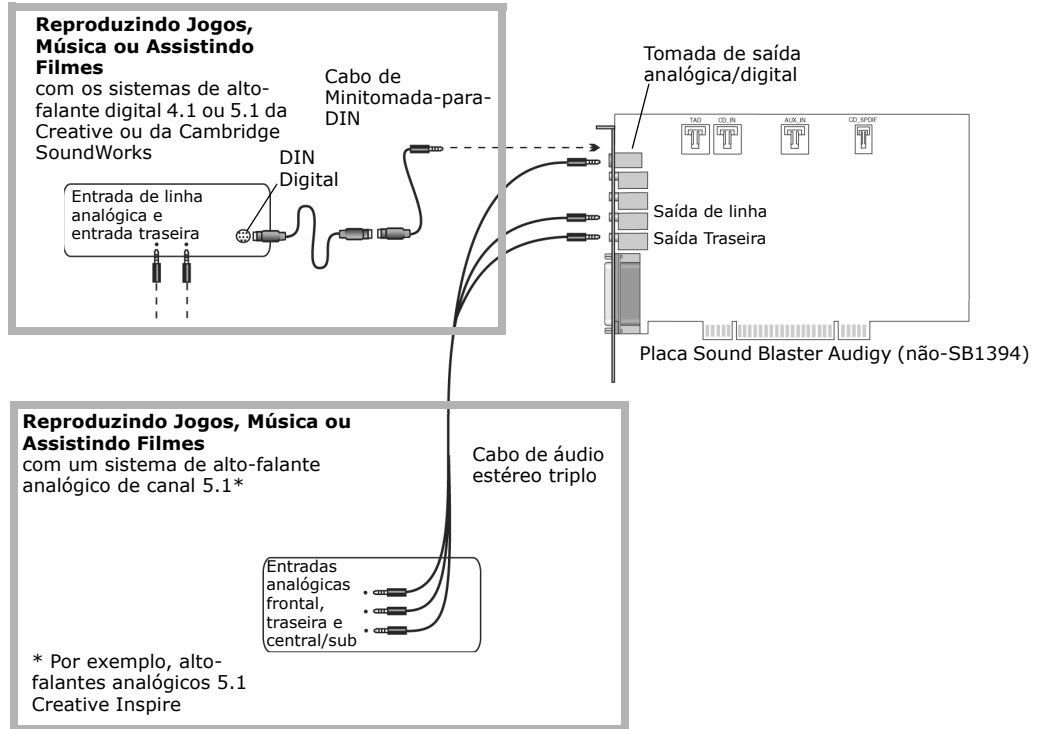
Figura 1-10: Conectando os sistemas de alto-falantes à placa Sound Blaster Audigy (não-SB1394).
