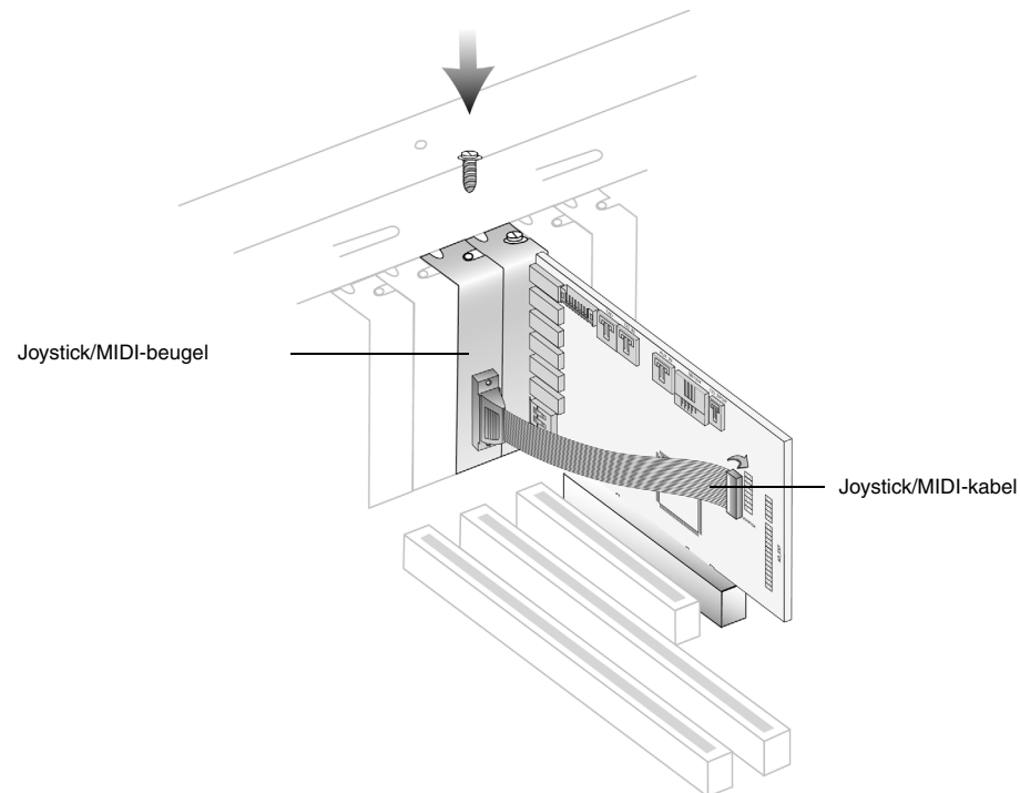
Afbeelding 1-5: De geluidskaart vastmaken aan de uitbreidingsleuf.
