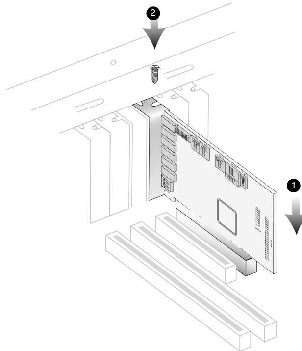
Afbeelding 1-4: De geluidskaart vastzetten in de uitbreidingsleuf.
