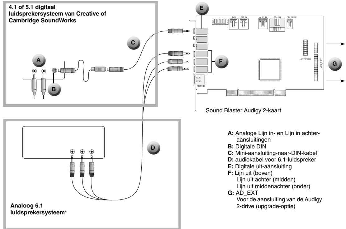
Afbeelding 1-8: De Sound Blaster Audigy 2-kaart aansluiten op luidsprekersystemen.
