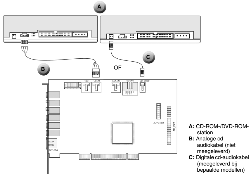
Afbeelding 1-6: Een analoge/digitale audiokabel aansluiten op een CD-ROM-/DVD-ROM-station.
