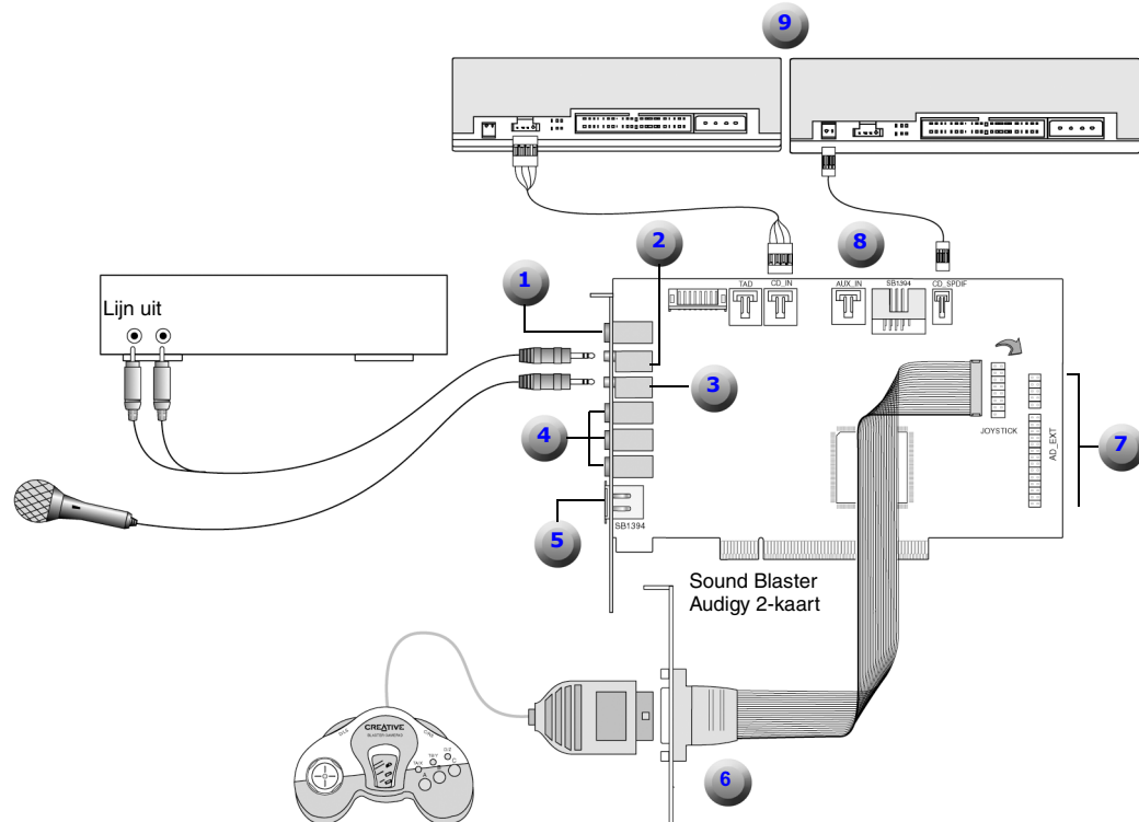
Afbeelding 1-7: Andere apparatuur aansluiten
