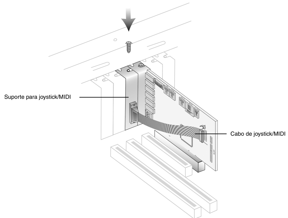
Figura 1-5: Prendendo a placa de áudio no slot de expansão.
