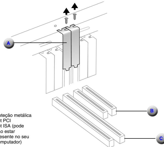
Figura 1-3: Removendo as peças metálicas
