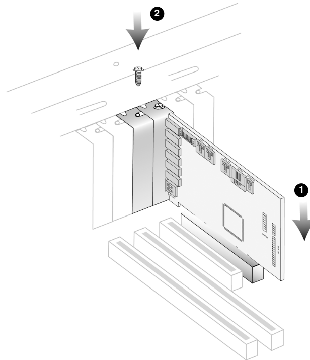
Figura 1-4: Prendendo a placa de áudio no slot de expansão.
