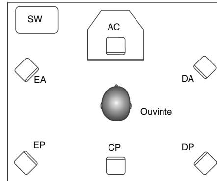
Figura 1-10: Posições recomendadas para os alto-falantes.
