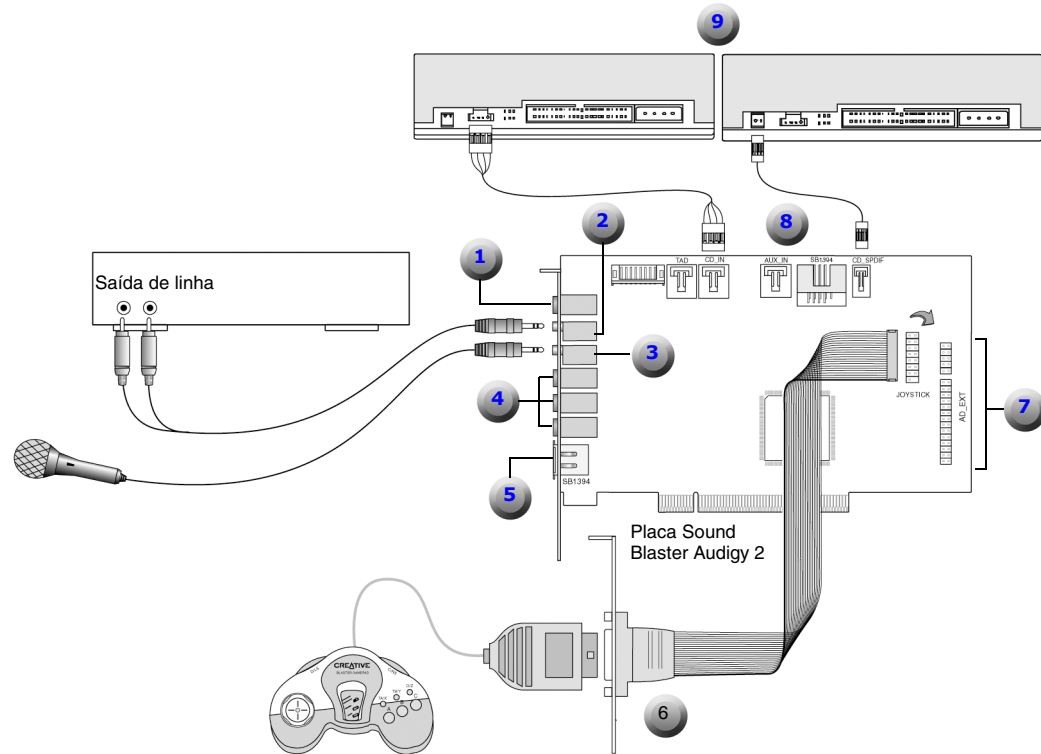
Figura 1-7: Conectando outros dispositivos
