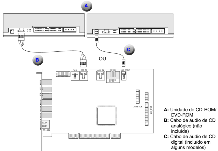
Figura 1-6: Conectando cabos de áudio analógico/digital às unidades de CD-ROM/DVD-ROM.
