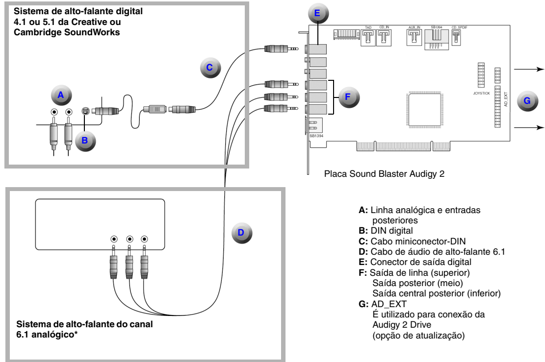
Figura 1-8: Conectando a placa Sound Blaster Audigy 2 aos sistemas de alto-falante.
